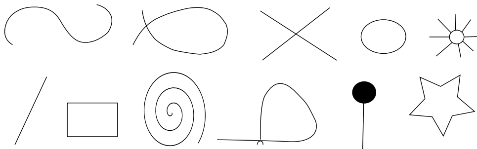
FIGURE 9.1 – Courbes ou pas courbes ?
