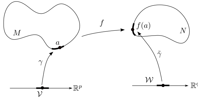
FIGURE 9.3 – Via les paramétrages, on ramène l'étude de la régularité à des fonctions définies sur des ouverts de \mathbb{R}^p .
