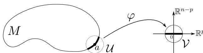
FIGURE 9.2 – \varphi « redresse » M au voisinage de a .
