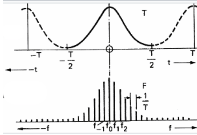
FIGURE 3.1. (Haut) Un signal régulier T -périodique réel F(t) , F : \mathbb{R} \rightarrow \mathbb{R} . (Bas) Module de ses coefficients |c_n| vs n = représentation fréquentielle de F . Notons la symétrie de |c_n| et aussi la décroissance de |c_n| lorsque n croît.
