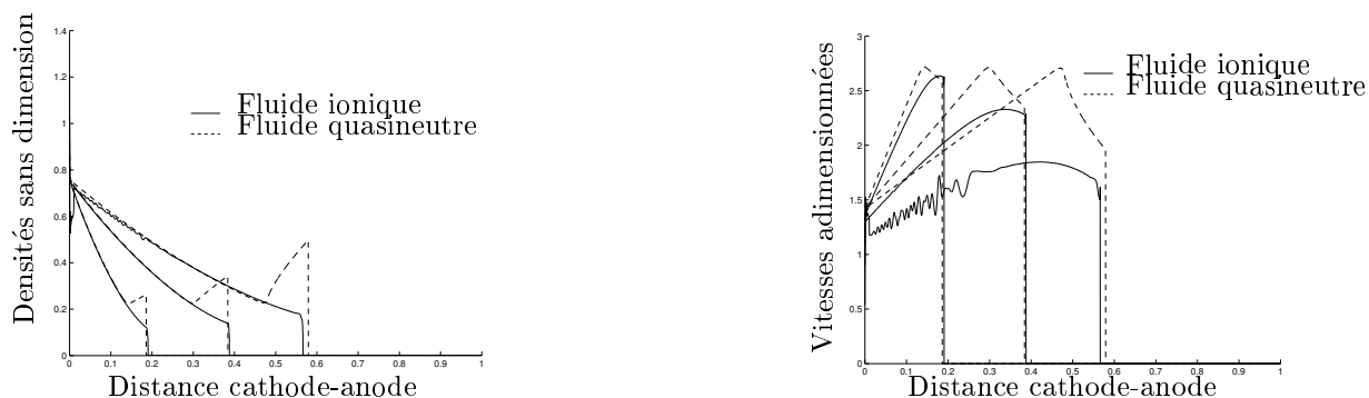
Figure 1: Densités et vitesses du fluide ionique issues du modèle bifluide comparées à la densité et à la vitesse du plasma du modèle quasineutre : quantités observées entre la cathode x = 0 et l'interface aux temps t = 0.07\tau , t = 0.15\tau , t = 0.24\tau .
