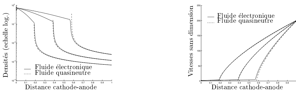
Figure 2: Densités et vitesse du fluide électronique issues du modèle bifluide comparées à la densité et à la vitesse du plasma issues du modèle de Child-Langmuir : quantités observées entre l'interface et l'anode x = 1 aux temps t = 0.07\tau , t = 0.15\tau , t = 0.24\tau .
